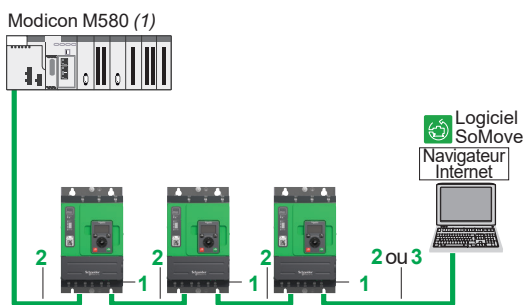
Démarrateur progressif ATS480 + module VW3A3720
